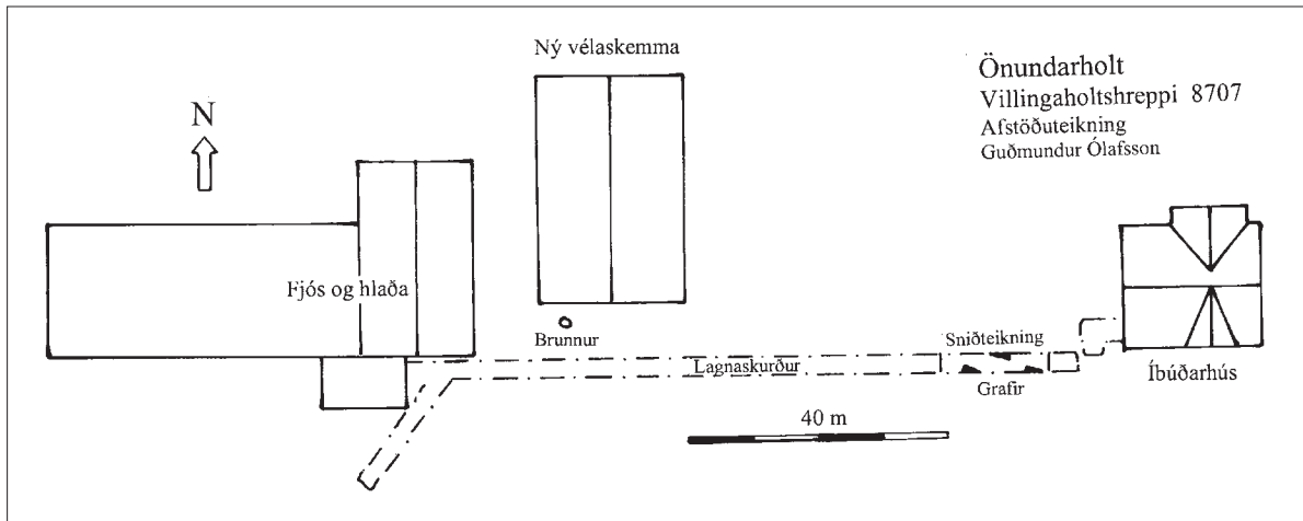
Afstöðuteikning af bæjarhúsum, lagnaskurði og vélahúsi.
