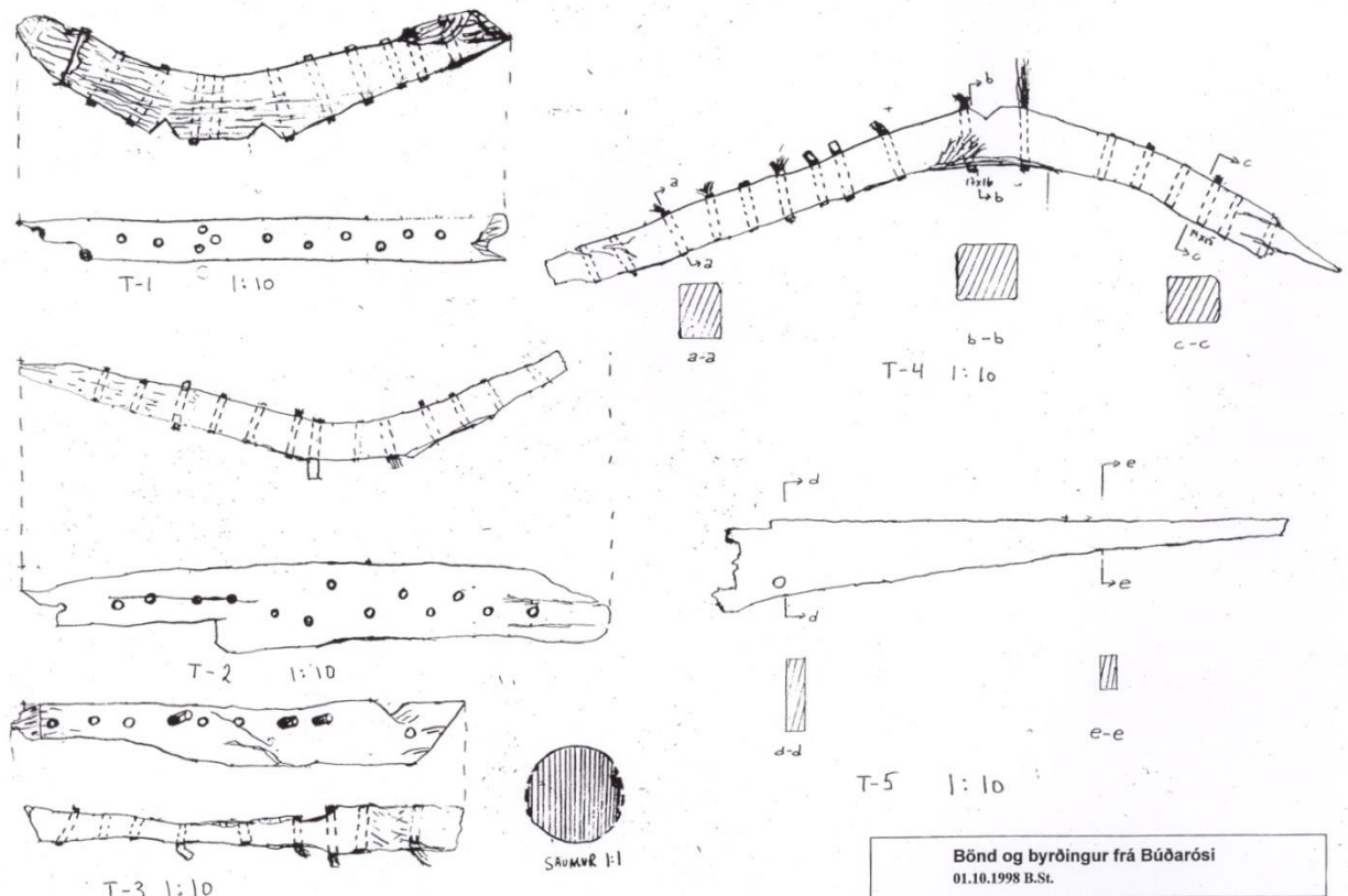
Mynd 4. Teikningar af skipaviðum. Teikningin er smækkuð niður um helming. (Teikn. Björn Stefánsson).
