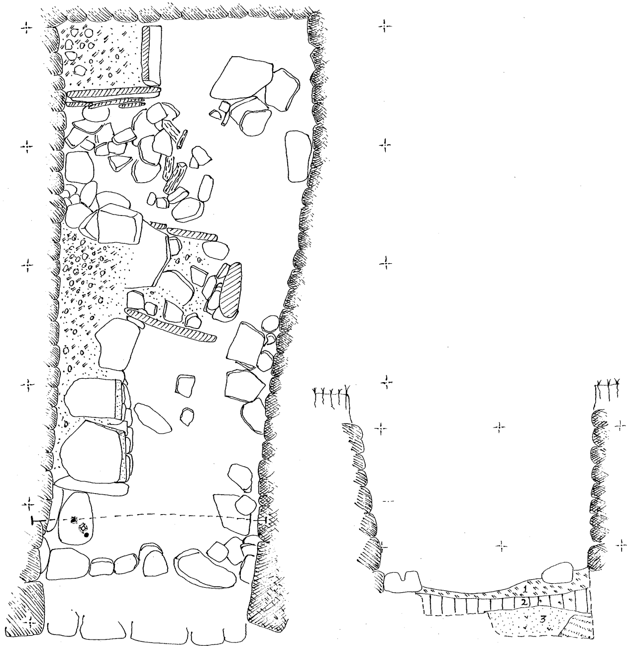
Flatar- og sniðteikning af smiðjunni á Keldum. Einn metri er á milli krossanna. (Teikn. G.Ó. og R.T.).
